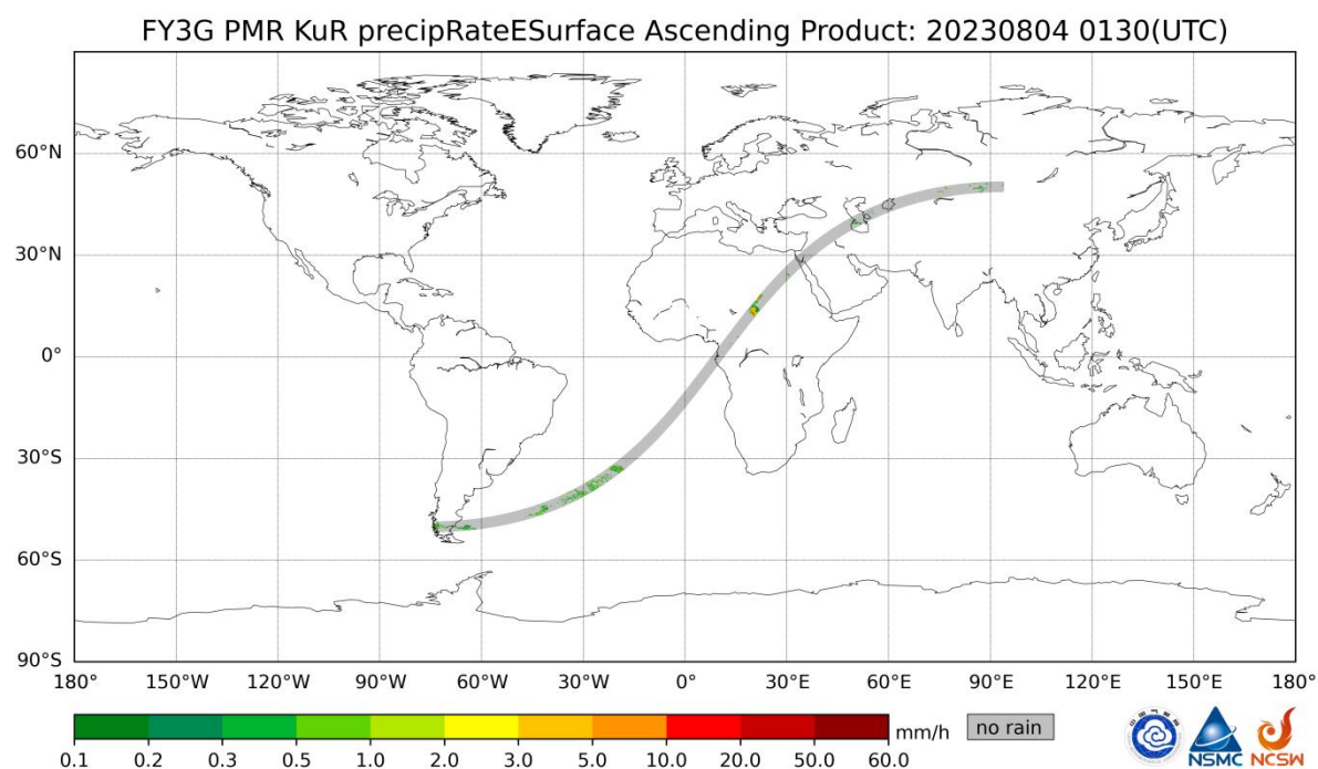
图 4-1 FY-3G PMR Ku 雷达升轨快视图
