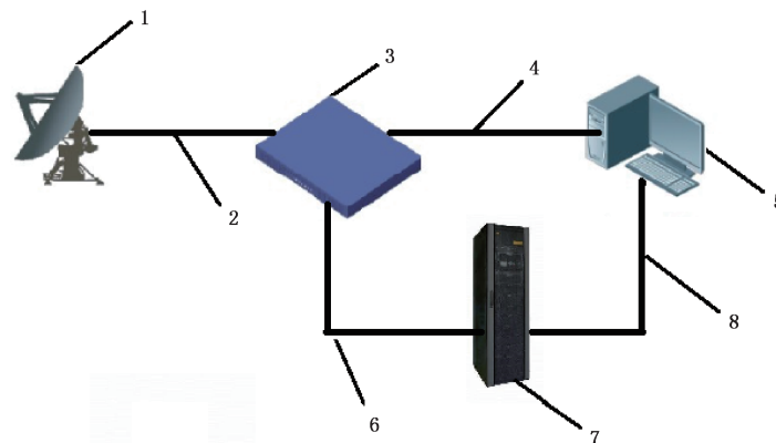
A.2 地基电离层闪烁观测仪器安装连接示意图
